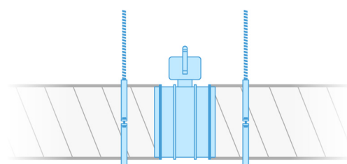
Installation entre deux gaines rigides
