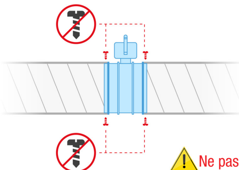
Installation entre deux gaines rigides
