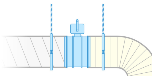
Installation entre deux gaines rigides
